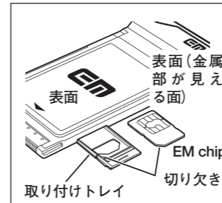
① EM chipの金属部を上向きにし、トレイの切り欠き部を合わせてください。
